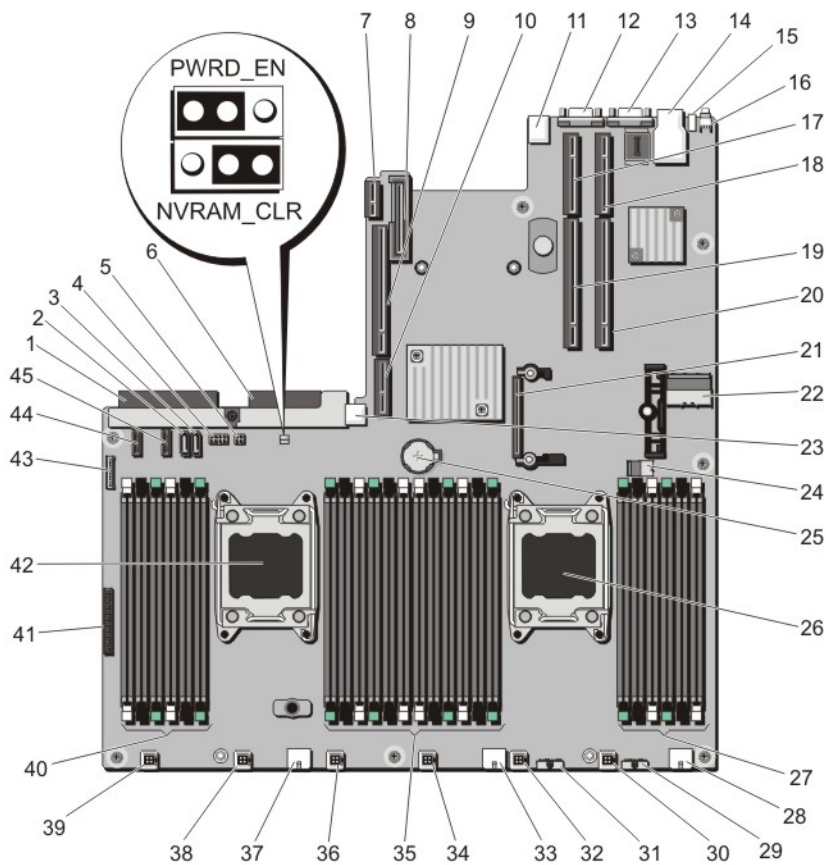
Ilustración 49. Puentes y conectores de la placa base
