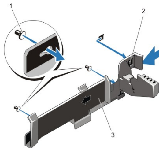
Ilustración 22. Extracción e instalación del soporte de retención de cables
