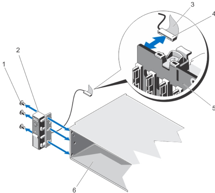
Ilustración 46. Extracción e instalación del panel de control
