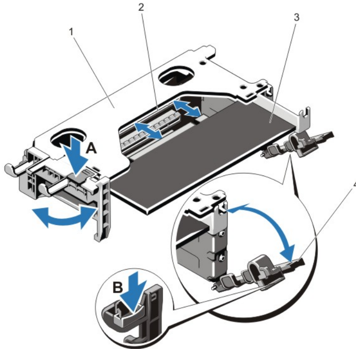
Ilustración 24. Extracción e instalación de la tarjeta vertical de expansión 1
