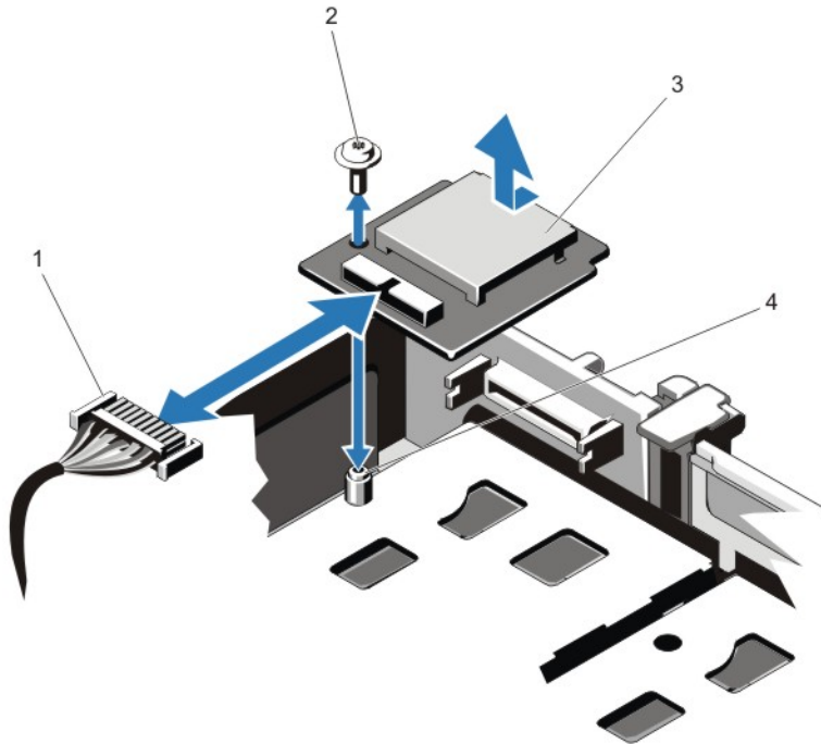
Ilustración 32. Extracción e instalación de una unidad de memoria vFlash
