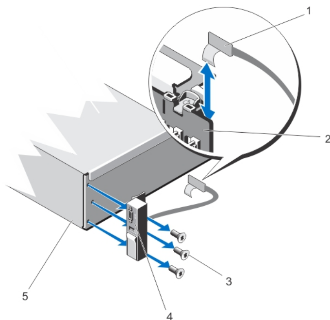
Ilustración 47. Extracción e instalación del ensamblaje del panel de E/S
