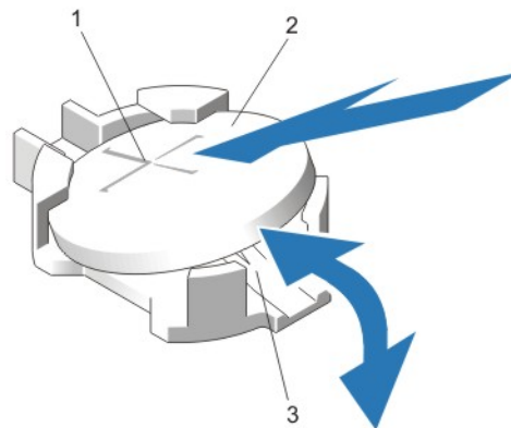
Ilustración 41. Sustitución de la pila del sistema
