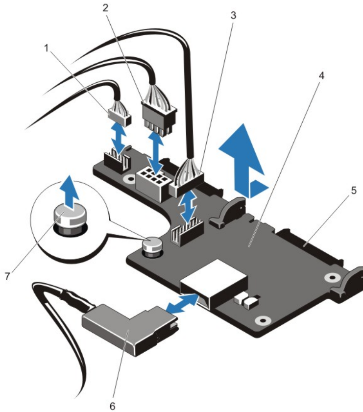
Ilustración 44. Extracción e instalación del plano posterior de la unidad de disco duro (x2) de 2,5 pulgadas (parte trasera)
