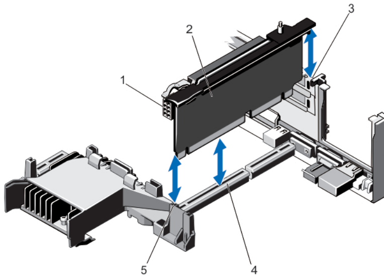
Ilustración 27. Extracción e instalación del soporte vertical 2 para tarjetas de expansión
