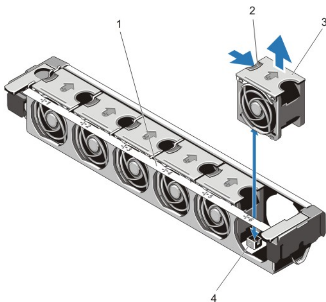
Ilustración 17. Extracción e instalación de un ventilador de refrigeración
