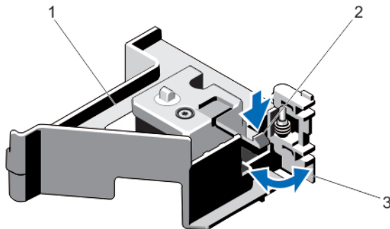
Ilustración 21. Apertura y cierre del pestillo del soporte de tarjeta PCIe
